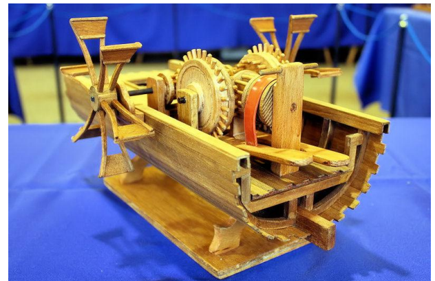
Barca a pedali
